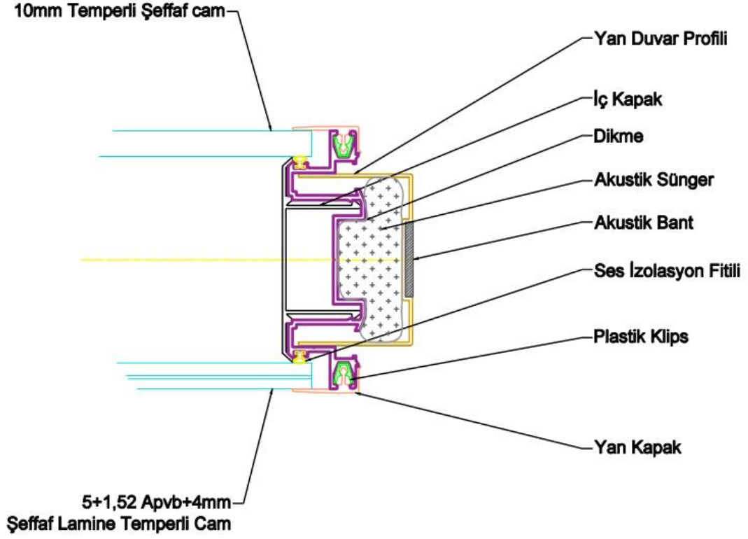
Şekil 3.2 Teknik Çizim 2
