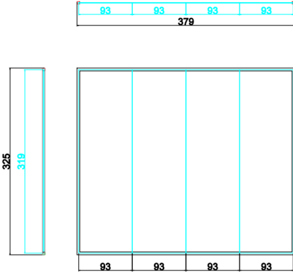
Şekil 3.1 Teknik Çizim 1
