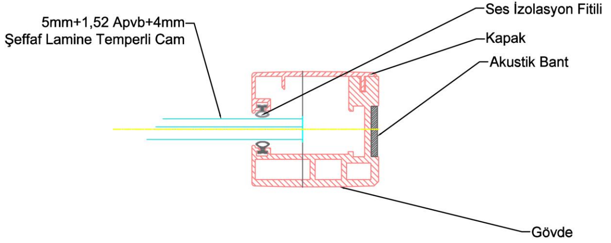
Şekil 3.2 Teknik Çizim 2
